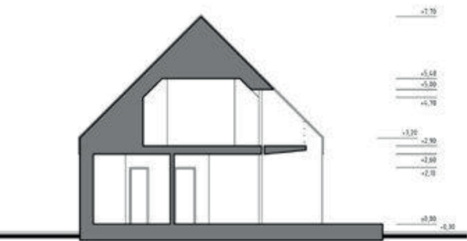
lõige A - A
